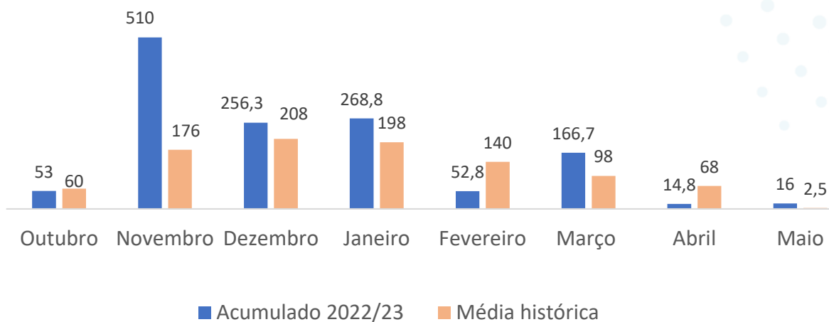
Precipitação mensal 2022/2023
